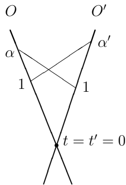
Rys. 4 Umowa \alpha = \alpha' stanowi o równouprawnieniu obserwatorów inercjalnych.
