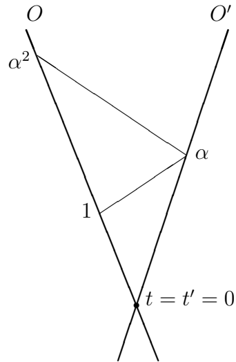
Rys. 5 Konsekwencja umowy i twierdzenia Talesa.
