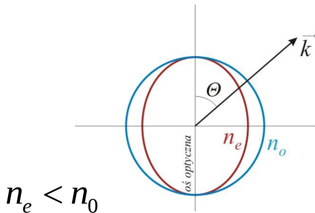
kryształ jednoosiowy ujemny
