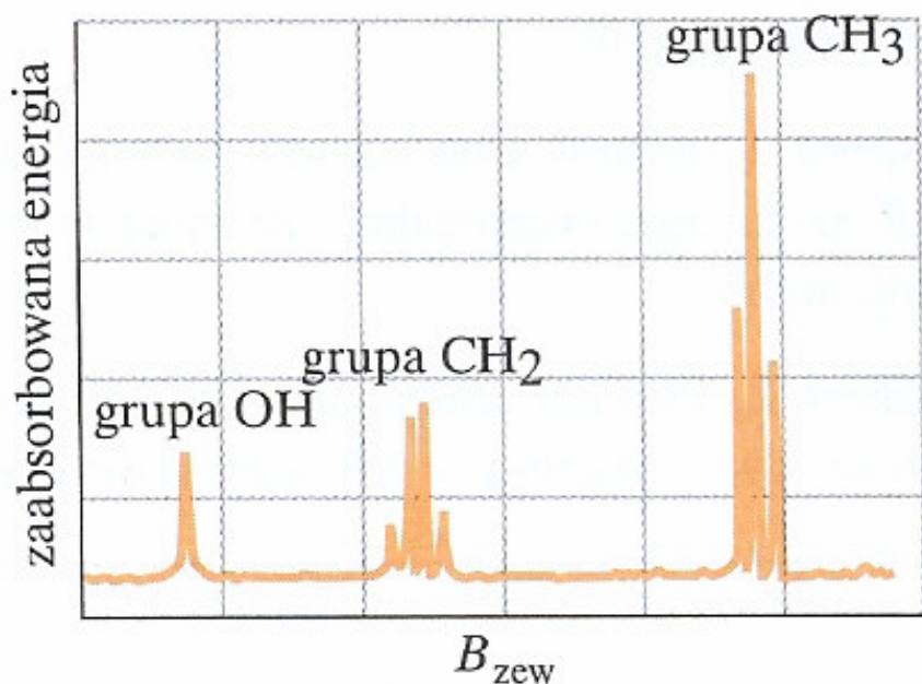
Widmo NMR dla etanolu
