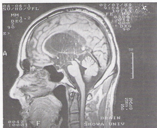
Ryc. 16.2. Przekrój strzałkowy głowy. Metoda FE, parametry: T_R = 300 ms, T_E = 14 ms, obraz zależny od T_1 , warstwa 5 mm, matryca 256 \times 256 , FOV 25 cm, 8 NAQ. Wodogłowic: ← komora mózgowa poszerzona, ► ciało modzelowate ścięzione. (1) gruczołowa część przysadki, (2) przedni płat przysadki, (3) nerw wzrokowy, (4) most, (5) wodociąg mózgu, (6) komora czwarta.
