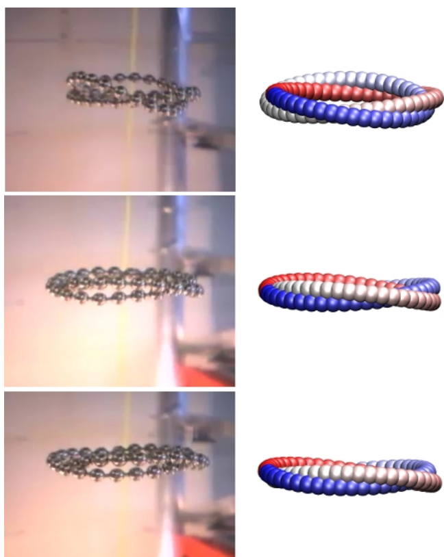
Zawężłone pętle opadające w lepkiej cieczy: eksperyment (z lewej) i symulacja komputerowa (z prawej). (Źródło: P. Szymczak, Wydział Fizyki UW)
