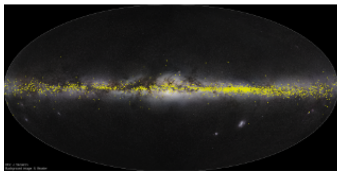
Cefeidy w Drodze Mlecznej (J. Skowron / OGLE, mapa Drogi Mlecznej autorstwa S. Brunier)
