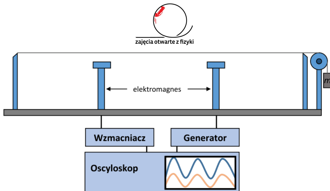
Rysunek 2. Schemat układu pomiarowego.
