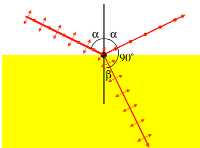
Rys. 13.20 Odbicie fali od dielektryka pod kątem Brewstera
