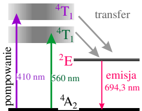
Rys. 14.19 Przejścia wewnątrz jonu chromu \text{Cr}^{3+} (w \text{Al}_2\text{O}_3 )
