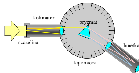
Rys. 14.15 Spektroskop przymatyczny
